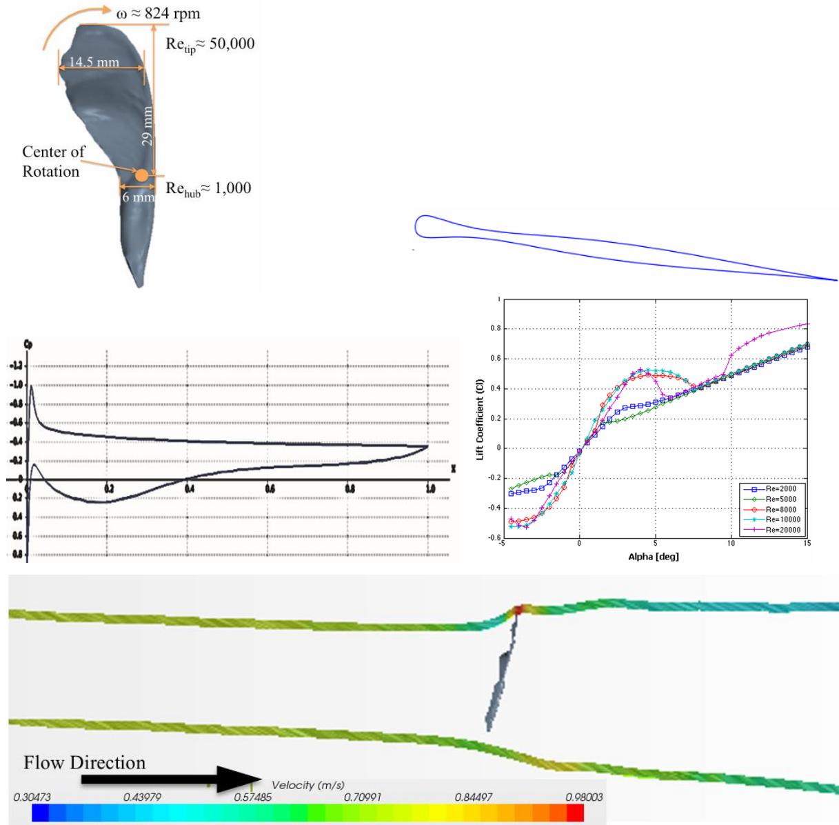
Şekil 7. Akçaağaç tohumu ve aerodinamik, tipik dönme hızı değeri, Reynolds sayısı, airfoil, Cp grafiği, Kaldırma katsayısı, CFD ile akçaağaç tohumu etrafındaki akış hızı [18].
