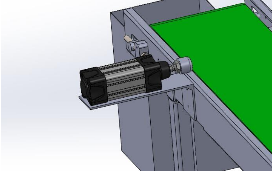
Görsel 1.2 Piston Bağlantı
