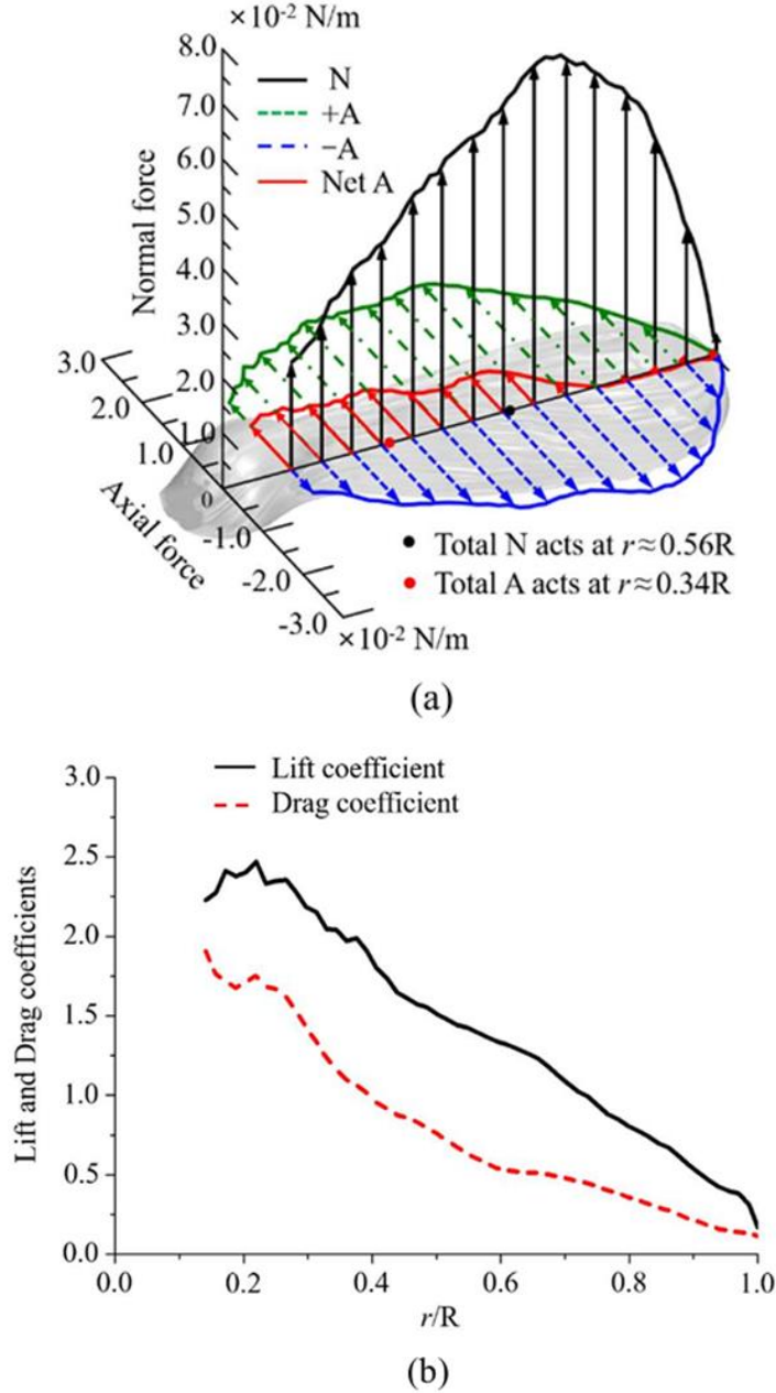
Şekil 12. Palmatum akçağaç tohumu için kuvvetlerin kanat açıklık(spanwise) yönünde dağılımı (a) normal ve eksenel kuvvetler (b) kaldırma ve sürüklenme katsayıları [21].
